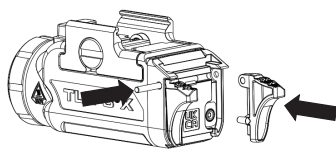
Schalter-Montage
